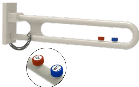
Anschluss verdeckt mit Montageplatte mit 1 E-Taster Connection to mounting plate with 1 E-Button
