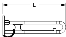
Anschluss verdeckt mit Montageplatte mit 2 E-Taster Connection to mounting plate with 2 E-Button
