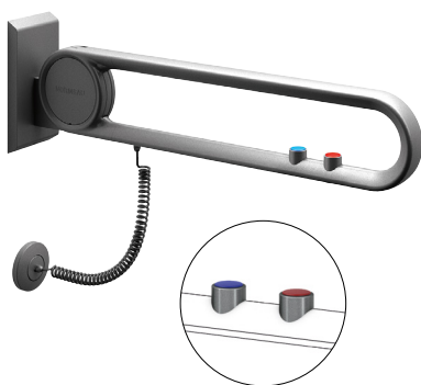
Aansluiting aan muur met 1 elektronische schakelaar Branchement mural avec un bouton de commande
