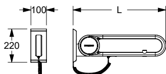
Aansluiting met montageplaat verdekt met 2 elektronische schakelaar Branchement mural avec deux boutons de commande
