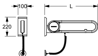
Aansluiting aan muur met 2 elektronische schakelaar Branchement mural avec deux boutons de commande
