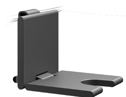
Einhängesitz Suspendable lift-up shower seat
