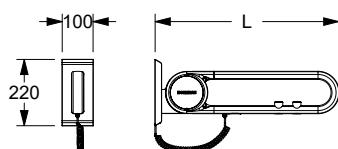
Anschluss verdeckt mit Montageplatte mit 2 E-Taster Connection to mounting plate with 2 E-Button
