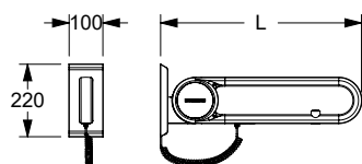
Anschluss verdeckt mit Montageplatte mit 1 E-Taster Connection to mounting plate with 1 E-Button
