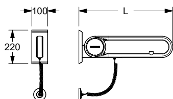
Wandanschluss mit 2 E-Taster Wall mounting with 2 E-Button
