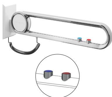
Anschluss verdeckt mit Montageplatte mit 1 E-Taster Connection to mounting plate with 1 E-button
