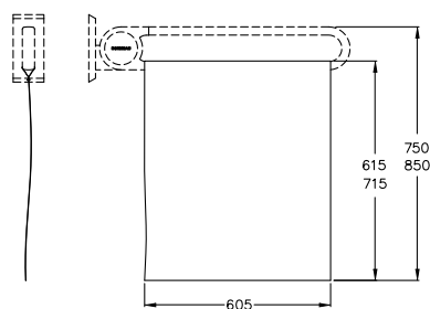
für Duschspritzschutz vario / for shower guard rail vario:
