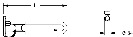
Anschluß verdeckt mit Montageplatte mit 2 E-Taster Connection to mounting plate with 2 E-Button
