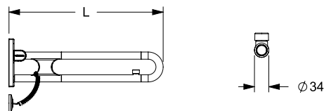
Aansluiting aan muur met 2 elektronische schakelaar Branchement mural avec deux boutons de commande
