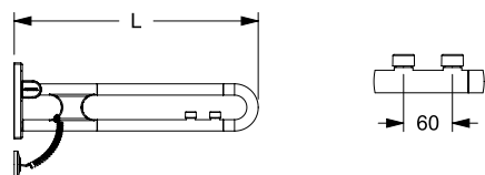
Aansluiting aan muur met 2 elektronische schakelaar Branchement mural avec deux boutons de commande
