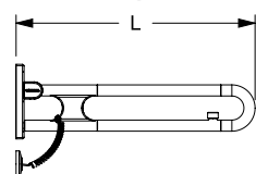
Wandanschluß mit 2 E-Taster Wall mounting with 2 E-Button
