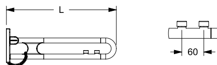
Anschluß vedeckt mit Montageplatte mit 2 E-Taster Connection to mounting plate with 2 E-Button
